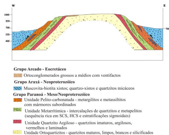
Figura 5 – Seção geológica esquemática representando um corte leste-oeste na porção central da Serra de Caldas.
