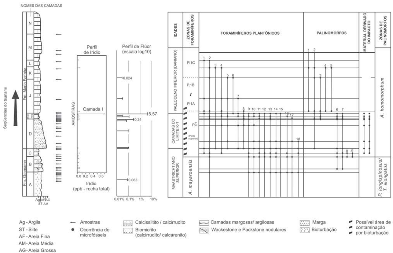
Figura 6 - Lito- e químioestratigrafias (irídio e flúor) e distribuição de microfósseis através da seção medida ao longo do limite K-T na pedreira Poty. Observar as anomalias de Ir e F em um argilito de 2-3cm de espessura (camada I, na parte superior da zona de foraminíferos plancônicos P.á). Foram utilizados os dados originais de foraminíferos de Koutsoukos (1996) e Albertão et al. (1994b), embora para a localização do limite K-T as camadas D a I sejam consideradas como as “camadas-limite”. Possíveis contaminações faunais abaixo de I são também consideradas. Foraminíferos plancônicos (análise de Eduardo A. M. Koutsoukos): (1) Woodringina hornestownensis ; (2) Guembeltria cretacea ; (3) Parasubbotina pseudobulloides ; (4) W. claytonensis ; (5) P. aff. pseudobulloides ; (6) Eoglobigerina eobulloides ; (7) Praemurica taurica ; (8) Parvularugoglobigerina eugubina ; (9) Pseudotextularia nuttalli ; (10) Pseudoguembelina costulata ; (11) P. palpebra ; (12) Rugoglobigerina ex gr. rugosa ; (13) R. scotti ; (14) Contusotruncana contusa ; (15) R. reicheli ; (16) Globotruncana aegyptiaca ; (17) Racemiguembelina fructicosa ; (18) Globotruncana falsocalcarata . Palinomorfos (análise de Marília P. S. Regali): (1) Proxapertites cursus ; (2) Pterospermopsis sp. ; (3) Veryhachium reductum ; (4) Schizeoisorites eocenicus ; (5) Echitriporites trianguliformis ; (6) Ariadnaesporites sp. ; (7) Dinogymnium spp. ; (8) Cricotriporites almadaensis ; (9) Crassitriapertites vanderhammeni .
