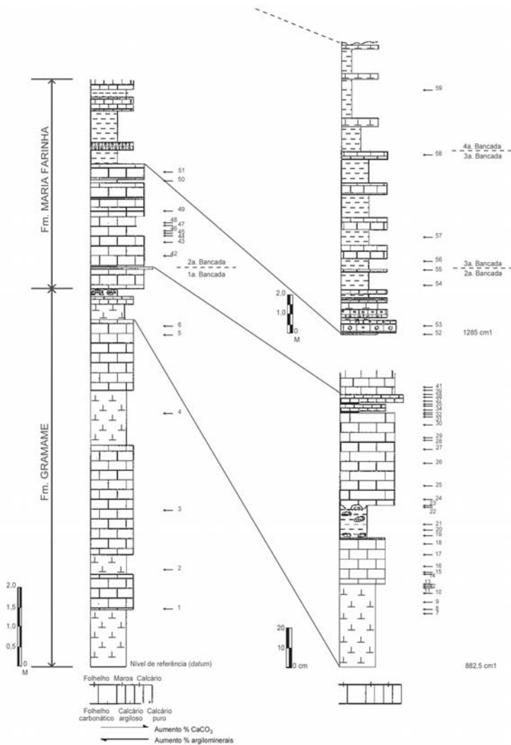
Figura 4 - Seção geológica esquemática da pedra Poty. As posições estratigráficas das amostras 1-59 estão indicadas. Detalhes da seção (parte inferior, lado direito da figura) são também mostrados na Fig. 6. Os símbolos litológicos são os mesmos da Fig. 6. Ver outros detalhes no texto.
