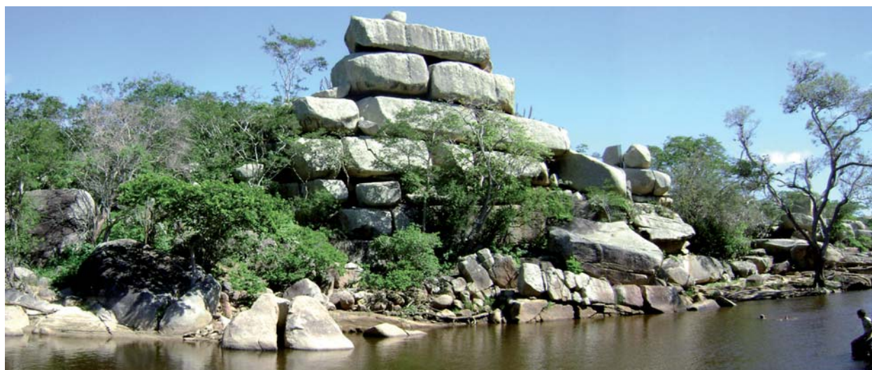
Figura 9 - Castle Koppie Saca de Lã apresentando ordem de fraturas ortogonais NS e EW e juntas de alívio encaixados em estrutura tipo riacho-fenda (falha transcorrente NNE sinistral). É possível observar que os blocos superiores estão vazados, permitindo o acesso sob estes.
