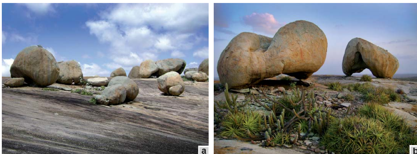
Figura 5 - (a) Visão de parte do Lajedo do Pai Mateus com seu característico “Mar de Bolas” formado por matacões de sienogranito. Ao centro da foto observa-se um bloco partido por processo de termoclastia; (b) Detalhe mostrando os dois mais famosos matacões da região, conhecidos como Boina e Pedra do Capacete, respectivamente;
