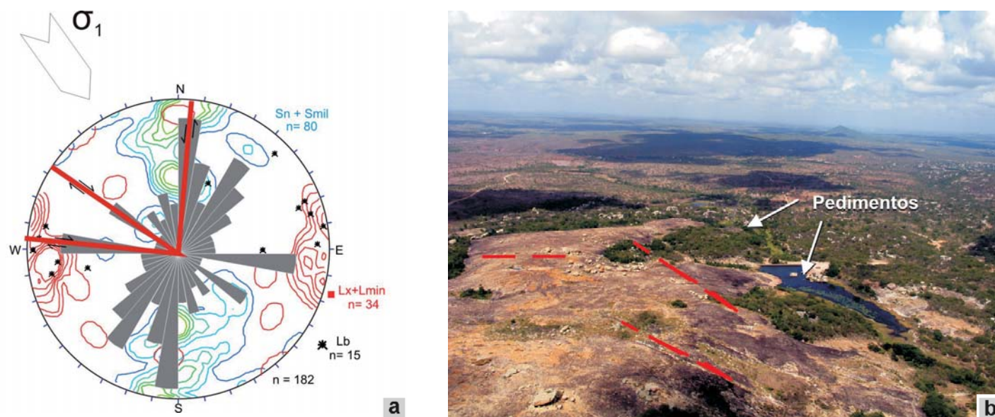
Figura 11 - (a) Diagrama sinóptico de igual área, hemisfério inferior para polos da foliação milonítica S_n + S_{mil} (linhas azuis e verde; isofrequência de valores: 1, 2, 3, 4 e 5) do entorno do Plutão Bravo; lineações de estiramento e mineral L_x + L_{min} e eixos de dobras L_b com sobreposição do conjunto de juntas, fraturas, falhas normais e transcorrentes rúpteis ( n=182 ) da área. As direções principais das faces dos blocos assimétricos (um lado mais alongado que o outro) coincidem em sua maioria com as direções N/NE e W/WNW; (b) Fotografia aérea do Lajedo do Pai Mateus apresentando alinhamento de blocos autóctones segundo direção aproximada NS e EW (Visada NNE).
