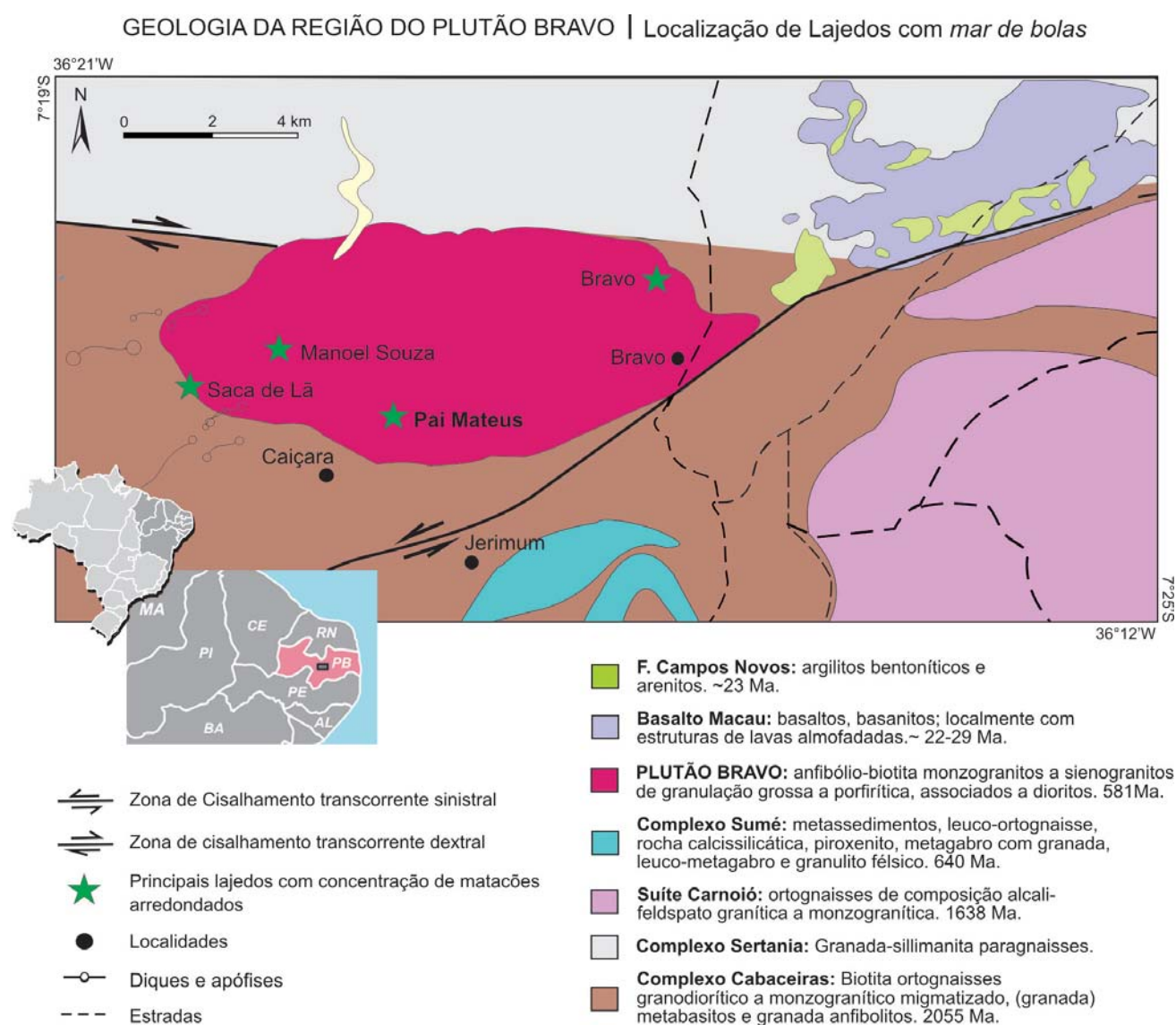
Figura 3 - Mapa geológico da área na qual se insere o Plutão Bravo e os principais lajedos portando campos de matacões (“mar de bolas”). É possível observar que os campos de matacões estão dispostos nas bordas da intrusão. Modificado de Lages & Marinho (2012).
