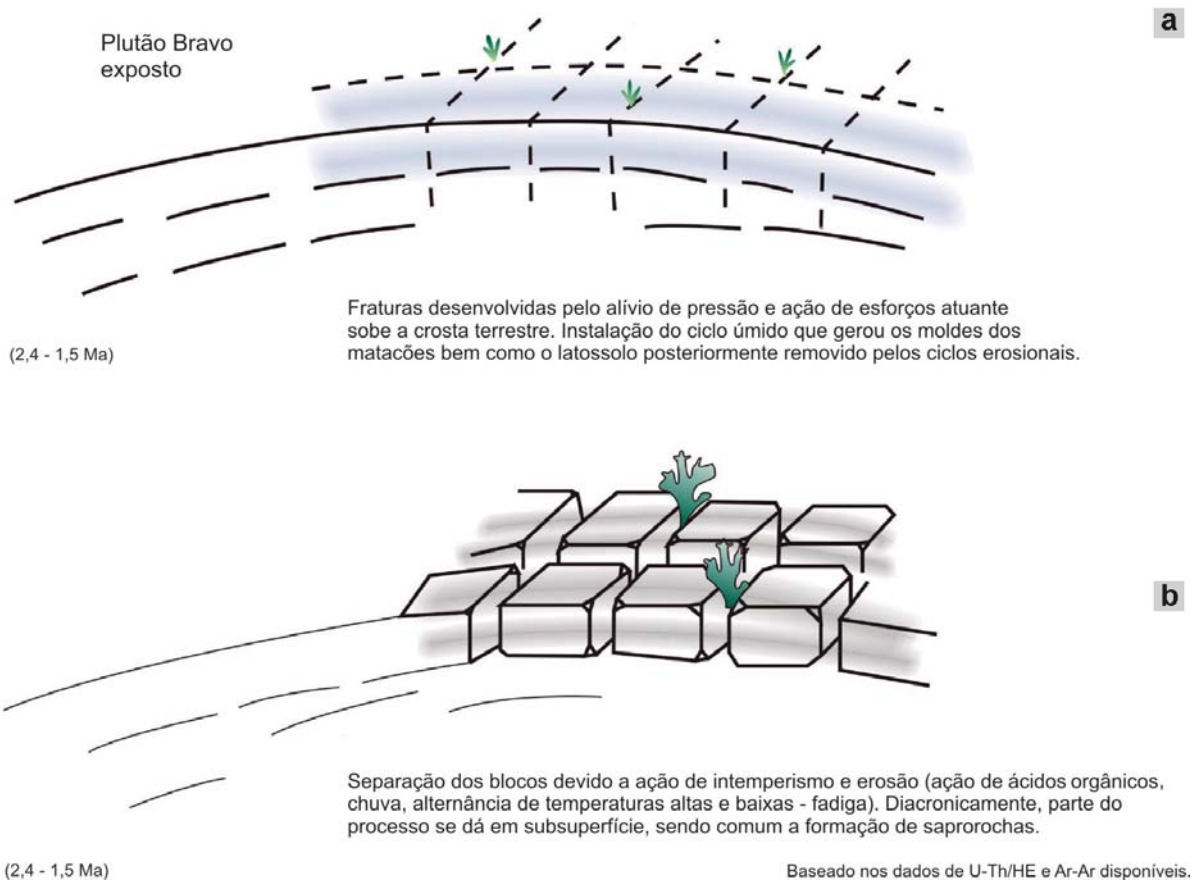
Figura 13 - (a) e (b) Evolução geológico-geomorfológica final observada atualmente na região do Plutão Bravo. Modificado a partir dos desenhos elaborados por Eduardo Bagnoli. Textos baseados nos métodos U-Th/He, Ar-Ar.
