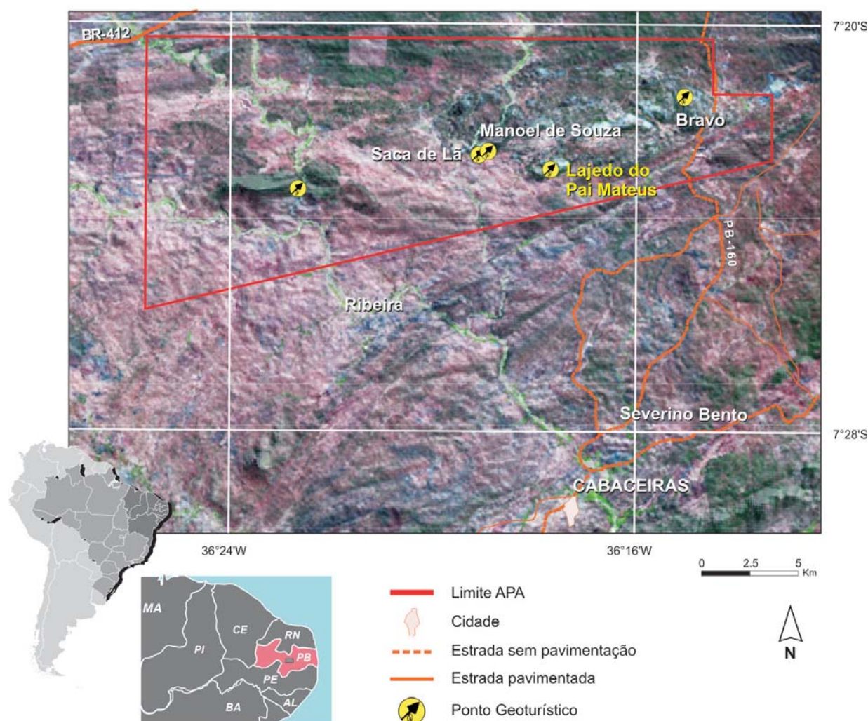
Figura 2 - Composição RGB 742 de cena obtida do Satélite Landsat sobre relevo sombreado, destacando o polígono da área de preservação da APA do Cariri Paraibano (Fialho et al. 2010), onde se insere o Plutão Bravo, que coincide com a área de preservação proposta para o Sítio SIGEP 068-Lajedo do Pai Mateus, além de outros pontos de interesse geoturístico. As principais cidades e vias locais de acesso estão representadas.
