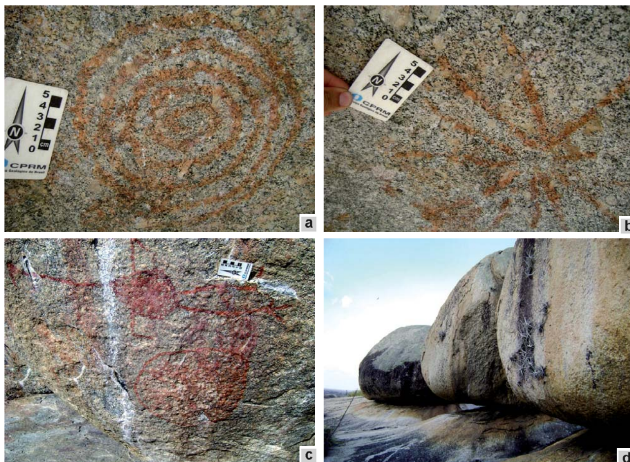
Figura 8 - (a) e (b) Representação de pintura rupestre com motivos “astronômicos” da Tradição Agreste, tais como espiral e o sol; (c) representação zoomórfica de uma ema com tamanho de cerca de 1 metro, animal que tem essa região como habitat; (d) alinhamento de matacões segundo sua posição original de emolduração em estágio de clima úmido, denota certo controle estrutural em diversas escalas de observação. Nota-se também, a erosão diferencial no lajedo que os abriga, pelo efeito da proteção que estes exercem sobre suas bases.
