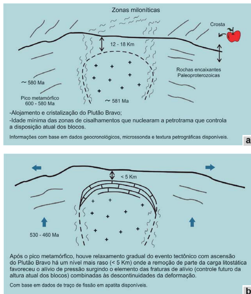
Figura 10 - (a) e (b) Evolução geológico-geomorfológica da região do Plutão Bravo, com base em dados geocronológicos, microsonda eletrônica, traço de fissão em apatita e petrográfico (minerais e texturais).
