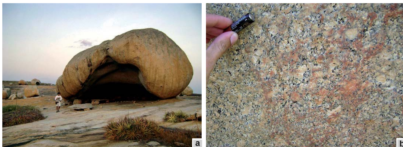
Figura 6 - (a) A Abrigo do “Pai Mateus” formado por cavidade abobadada de um matacão, onde a tradição oral diz ter vivido o Pai Mateus – um curandeiro ermitão do século XVIII. A maior parte das cavidades deste tipo tem suas aberturas voltadas para o oeste; (b) marca de mão espalmada impressa em face polida de bloco com tinta ocre à base de óxido de ferro.
