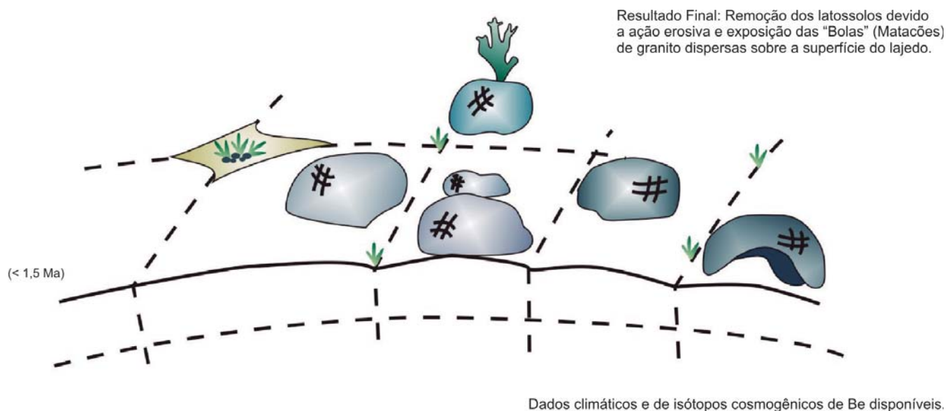
Figura 14 - Evolução geológico-geomorfológica final observada atualmente na região do Plutão Bravo. Modificado a partir dos desenhos elaborados por Eduardo Bagnoli. Textos baseados nos métodos de isótopos cosmogênicos de Be e dados de climatologia.
