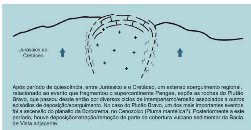
Figura 12 - Evolução geológico-geomorfológica da região do Plutão Bravo, com base em dados geocronológicos, microsonda eletrônica, traço de fissão em apatita e petrográfico (minerais e texturais).
