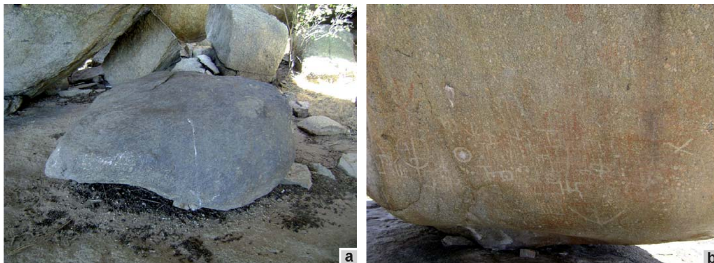
Figura 7 - (a) Lajota natural sob abrigo de matacão abobadado com face superior exibindo brilho, dado o intenso polimento a que foi submetida, que certamente foi de serventia ao homem pregresso; (b) Inscrições rupestres em tinta ocre de figuras da Tradição Agreste, em inédita associação com inscrições em baixo relevo do tipo Itacoatiaras em matacão com face polida no lajedo do Sítio Bravo. Nota-se que alguns motivos se encontram parcialmente vandalizados/degradados.
