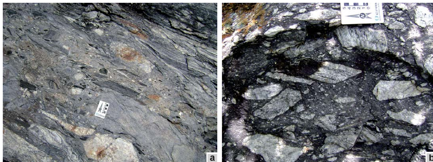
Figura 4 - (a) Textura protoclástica no contato entre rochas graníticas do Plutão Bravo e o ortogneisse encaixante (ortognaissificação); (b) Brecha plutônica com matriz diorítica portando xenólitos da rocha ortognaissica encaixante.
