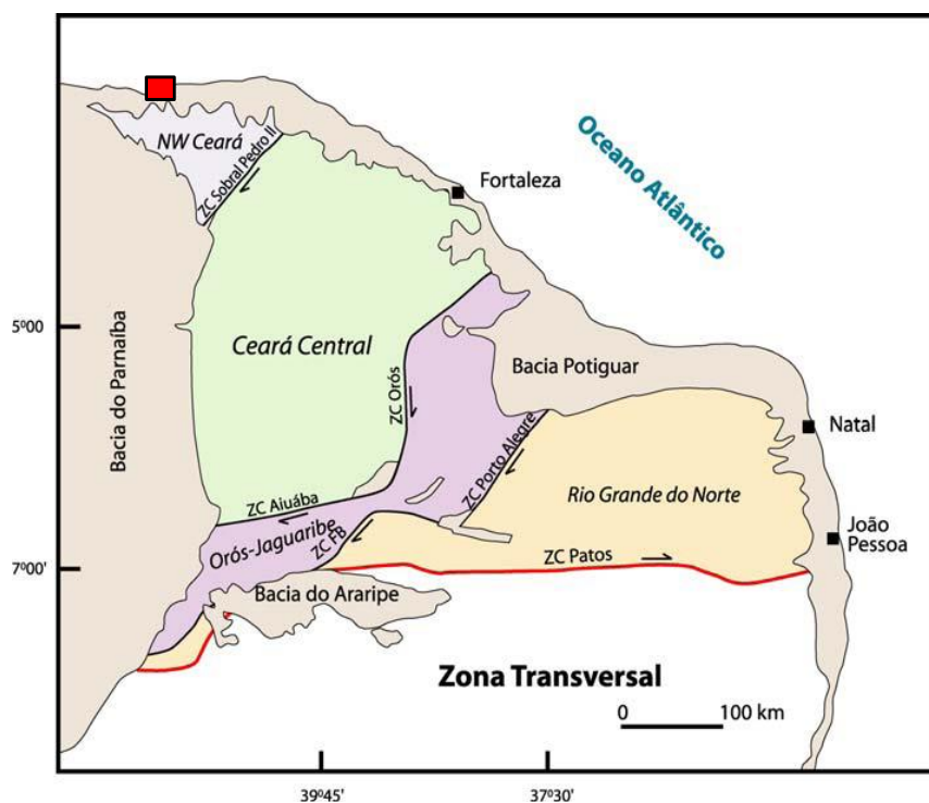
Figura 3 – Domínios geológicos (Rio Grande do Norte, Orós-Jaguaribe, Ceará Central, NW do Ceará) da porção Setentrional da Província Borborema e localização da área em estudo (Fonte: Cavalcante et al. , 2003).
