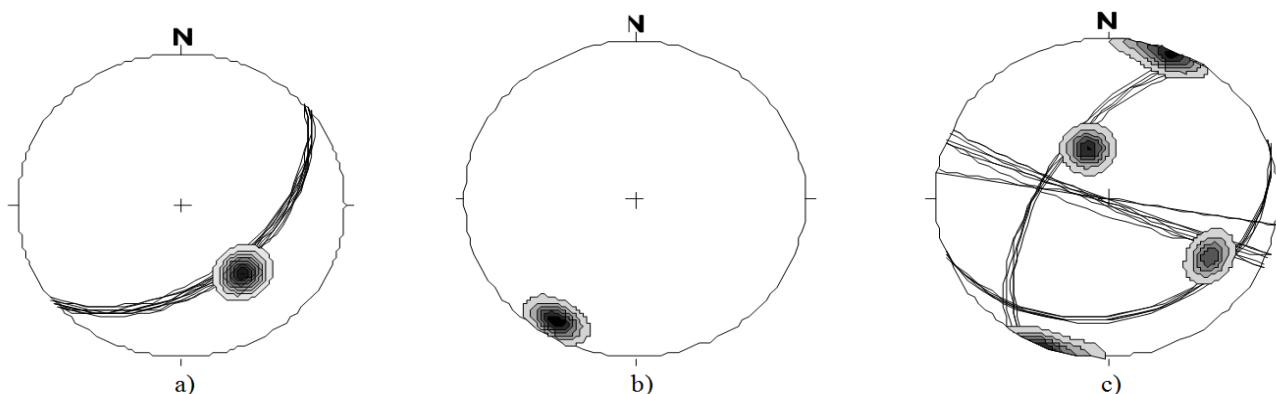
Figura 13 – a) Estereogramas da foliação S 1 e dos paleoplanos de acamamento S 0 mostrando mergulho preferencial para SE e direção NE (22 medidas); b) Estereograma da lineação de estiramento e de eixo de dobras paralelas e com caimento suave para SW (L xn // L bn ); c) Estereograma dos planos de fraturas existentes no afloramento da Pedra Furada, máximos obtidos a partir do pólo dos planos; os planos de fraturas (medida Clar) posicionam os tensores δ 1 na direção NE e δ 3 a SE.
