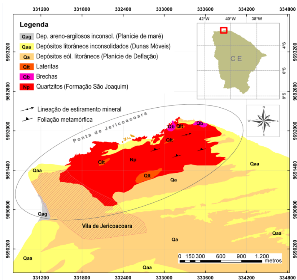
Figura 11 – Mapa geológico simplificado da área. Figure 11 – Simplified geologic map of the area.
