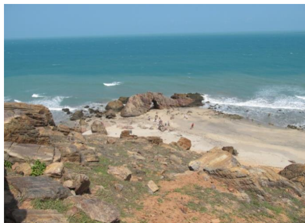
Figura 6 – Quartzitos e blocos soltos de coloração preta avermelhada (quartzitos ferruginosos).
