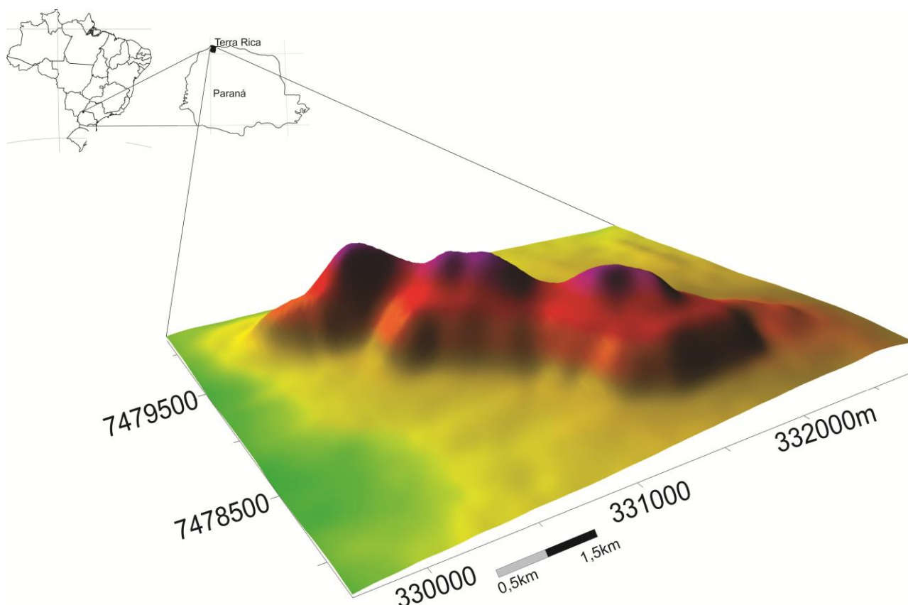
Figura 2: Localização regional e modelo de elevação de terreno dos Três Morrinhos. Figure 2: Três Morrinhos Hill location and terrain elevation model.
