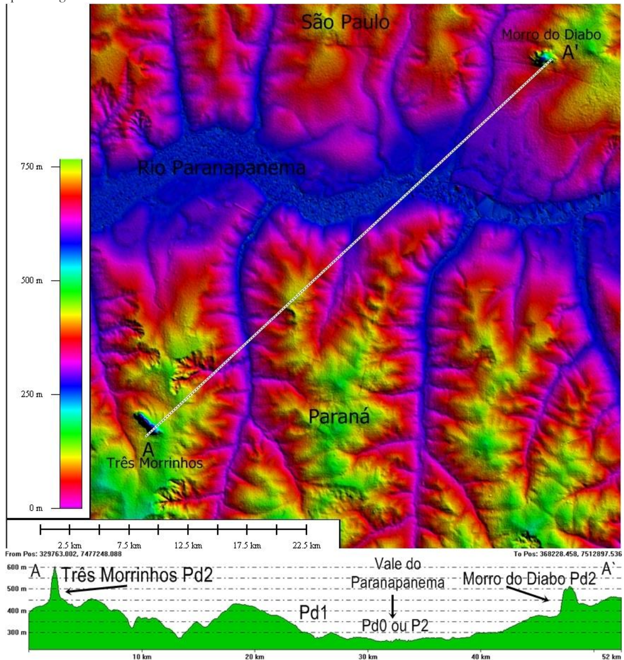
Figura 14: Seção topográfica transversal entre os Três Morrinhos (Terra Rica, Paraná) e o morro do Diabo (Parque Estadual Morro do Diabo, Teodoro Sampaio, São Paulo). Dados topográficos de imagens SRTM, Projeto TOPODATA-INPE.
