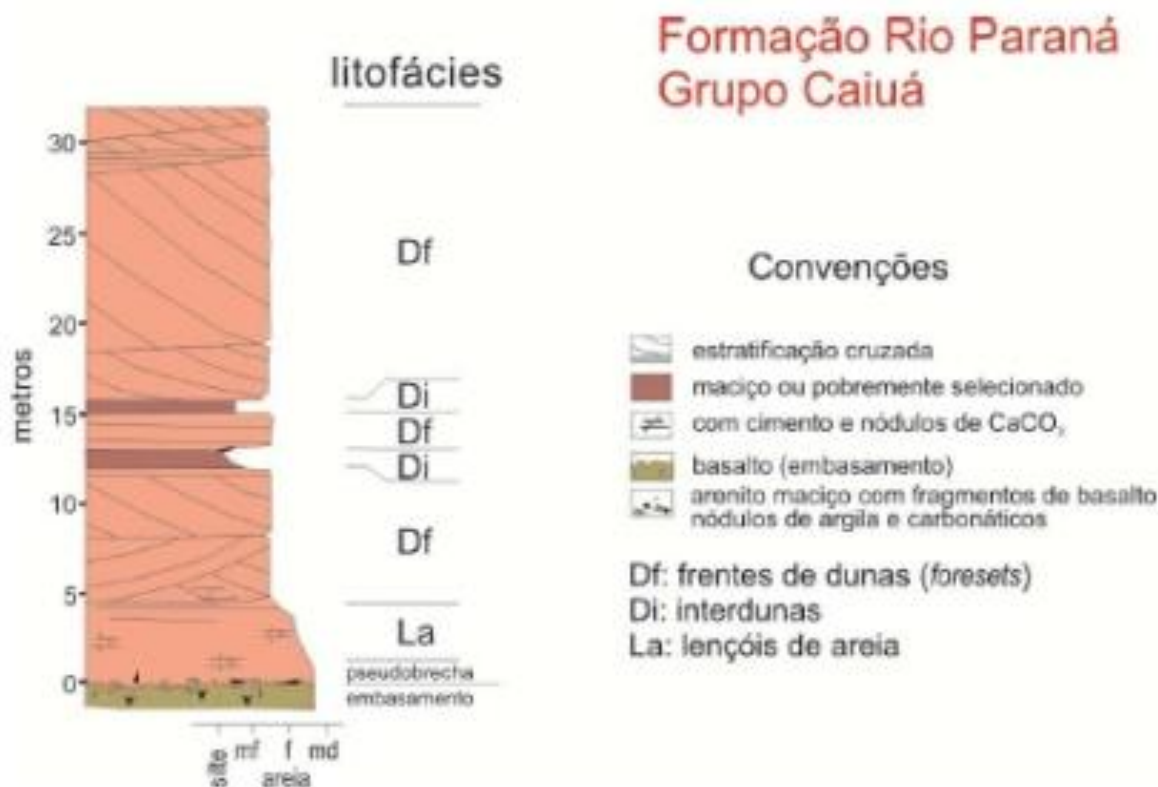
Figura 9: Seção-tipo da Formação Rio Paraná, com principais características da unidade, tipos de depósitos e contexto deposicional (dunas e interdunas eólicas). Definida na eclusa da U.H.E. Porto Primavera (Eng. Sérgio Motta), Pontal do Paranapanema (SP) e grandes exposições nas barrancas do rio Paraná.
