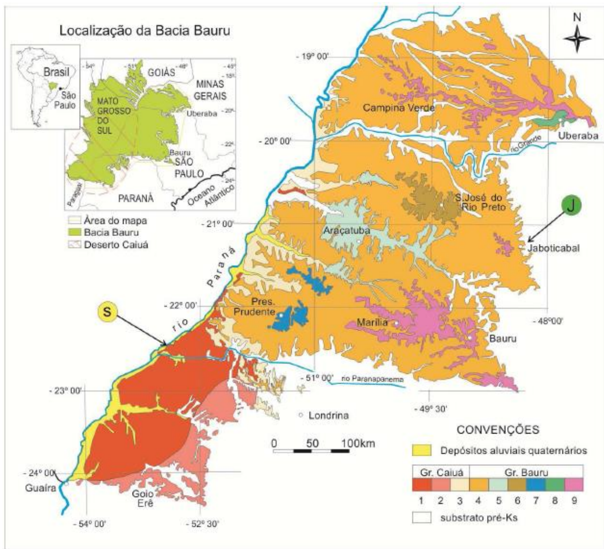
Figura 5: Mapa geológico da parte oriental da Bacia Bauru. Convenções: 1. Fm. Rio Paraná, 2. Fm. Goio Erê, 3. Fm. Santo Anastácio, 4. Fm. Vale do Rio do Peixe, 5. Fm. Araçatuba, 6. Fm. São José do Rio Preto, 7. Fm. Presidente Prudente, 8. Fm. Uberaba, 9. Fm. Marília. J=rocha alcalina de Jaboticabal, S=sismitos de Porto Primavera.
