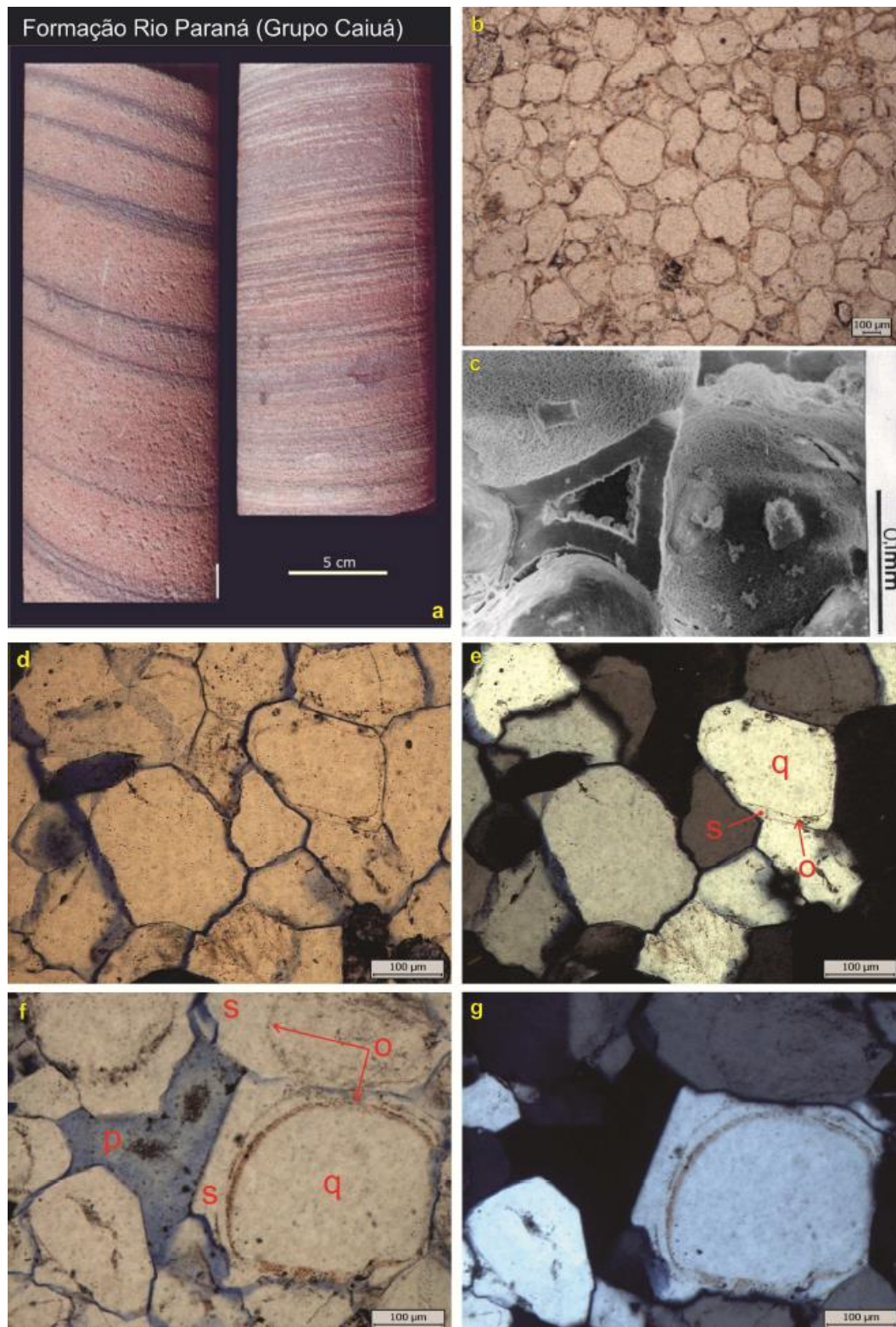
Figura 11: a. Estratificação cruzada, laminação e cores características dos arenitos da Fm. Rio Paraná, quando não silicificados; de testemunhos de sondagem da UHE Porto Primavera (SP); b. aspecto comum dos arenitos dos Três Morrinhos, exibindo grãos arredondados bem selecionados, com intensa cimentação por sílica, fotomicrografia com polarizadores descruzados; c. grãos arredondados de quartzo, com poros parcialmente preenchidos por cimento de sílica, imagem de MEV (elétrons secundários); d. aspecto de mosaico (faces mais retilíneas) dado pela silicificação intensa, que oblitera os poros originais dos quartzarenitos dos Três Morrinhos, fotomicrografia com polarizadores descruzados; e. mesma cena de d , com polarizadores cruzados, ( s ) é crescimento secundário (ou sintaxial) de sílica, ( o ) é película de óxidos/hidróxidos de Fe e Mn, pré-cimentação por sílica, ( q ) grão de quartzo; f. detalhe de quartzarenito com grãos arredondados de quartzo ( q ), revestido por película de de óxidos/hidróxidos de Fe e Mn ( o ) e posteriormente por sílica secundária, em duas fases ( s ), fotomicrografia com polarizadores descruzados; g. mesma cena de f , com polarizadores cruzados.
