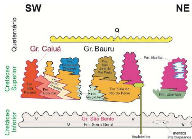
Figura 6: Carta estratigráfica da sequência neocretácea (segundo Fernandes & Coimbra 2000a).
