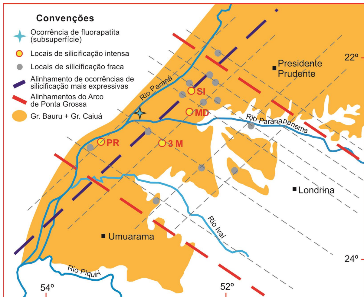
Figura 1: Locais de ocorrência de arenitos silicificados na porção meridional da Bacia Bauru. As mais importantes: 3M Três Morrinhos (PR); MD , Morro do Diabo (SP); SI , morro da fazenda Santa Ida (SP) e PR , morro da fazenda Porto Rico (margem esquerda do rio Paraná, PR).
