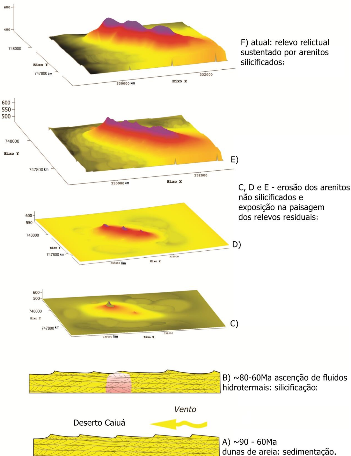
Figura 13: Modelo de evolução geomorfológica regional, para os Três Morrinhos e morro do Diabo. C, D, E e F foram geradas com o método de Seppômen, que permite a reconstituição de paleossuperfícies por meio de pontos de maior cota altimétrica, de forma irregular por quadrantes. Com aumento da área do quadrante tem-se nivelamento dos topos e assim a reconstituição das paleossuperfícies. Aplicações em geologia foram apresentadas por (Motoki et al. , 2008) e em geomorfologia por (Couto et al. , 2012) por meio de geoprocessamento.
