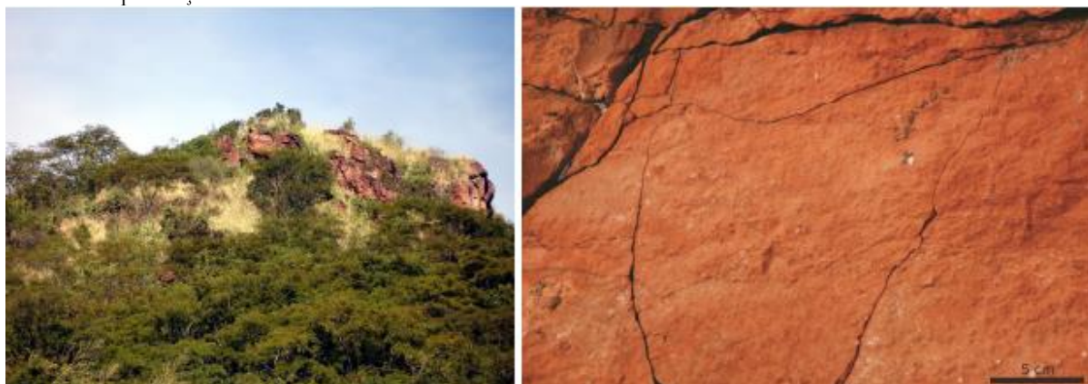
Figura 10: Arenito silicificado em exposições de superfície, lajes ou paredões nas encostas dos morros. A rocha apresenta aspecto em geral maciço, cor marrom alaranjado a rosado.
