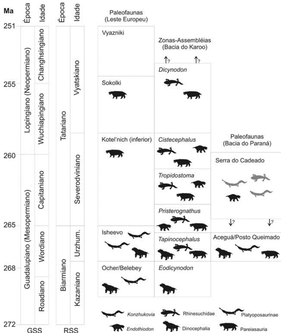
Figura 7 – Faunas de tetrápodes da Formação Rio do Rasto e correlação destas com as assembléias da Bacia do Karoo e da Plataforma Russa. Correlação entre o GSS (Global Stratigraphic Scale) e o RSS (Regional Stratigraphic Scale) do Leste Europeu baseada em Menning et al. (2006) e Resolutions (2006). Posicionamento das faunas cisuralianas em relação ao RSS baseado em Sennikov (1996), Golubev (2000), Modesto & Rybczynski (2004) e Tverdokhlebov et al. (2005). Correlação das Zonas-Assembléia do Grupo Beaufort com as faunas cisuralianas baseada em Rubidge (2005, 2007), Cisneros et al. (2005) e Lucas (2006). Siluetas baseadas em Cisneros et al. (2005); registros incertos em cinza.
