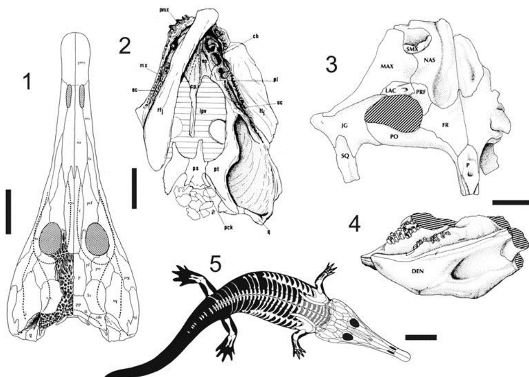
Figura 6 – Tetrápodos da Serra do Cadeado. (1) Crânio de Australerpeton cosgriffi em vista dorsal (retirado de Barberena, 1998); (2) crânio do temnosspôndilo brevirostre em vista palatal (retirado de Barberena & Dias, 1998); (3) crânio de Endothiodon em vista oblíqua dorsal-esquerda (retirado de Barberena & Araújo, 1976); (4) ramos mandibulares de Endothiodon em vista lateral esquerda (retirado de Barberena & Araújo, 1976); (5) reconstituição esquelética de A. cosgriffi , baseado em Barberena (1998) e Dias & Schultz (2003). Escalas = 5 cm (1-4); 15 cm (5).
