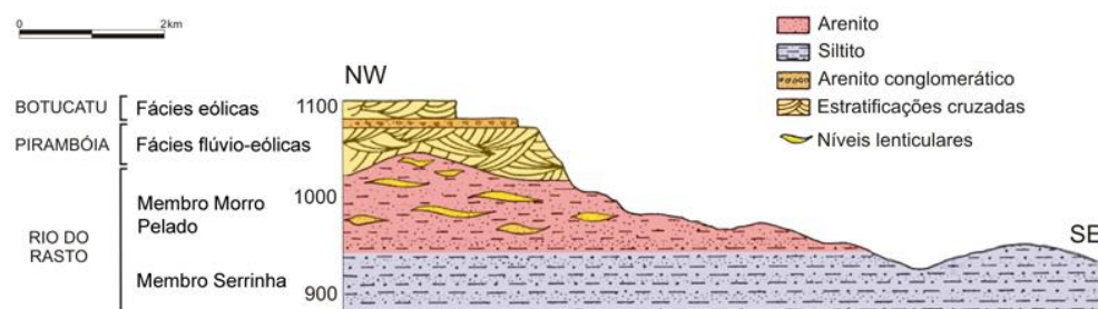
Figura 4 – Seção geológica esquemática da Serra do Cadeado (modificada de Barberena et al. , 1980). As inúmeras falhas geológicas e diques de diabásio da região não estão representados.
