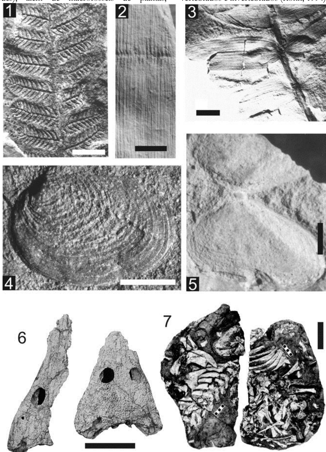
Figura 5 – Fósseis da Serra do Cadeado. (1) Pina de Pecopteris cadeadensis (Foto: Rosemarie Rohn); (2) fragmento de caule de Paracalamites (Foto: Rosemarie Rohn); (3) caules e folhas de Schizoneura gondwanensis (retirado de Cazzulo-Kleipzig & Correia, 1981); (4) valvas de Liograptus sp. (Foto: Rosemarie Rohn); (5) valvas articuladas de Terraia sp. (Foto: Rosemarie Rohn); (6) crânios parciais de Australerpeton cosgriffi em vista dorsal (retirado de Dias & Schultz, 2003); (7) esqueleto pós-craniano de A. cosgriffi (retirado de Dias & Schultz, 2003). Escalas = 1,5 cm (1), 1cm (2-3), 0,1 cm (4), 0,5 cm (5), 10 cm (6-7).
