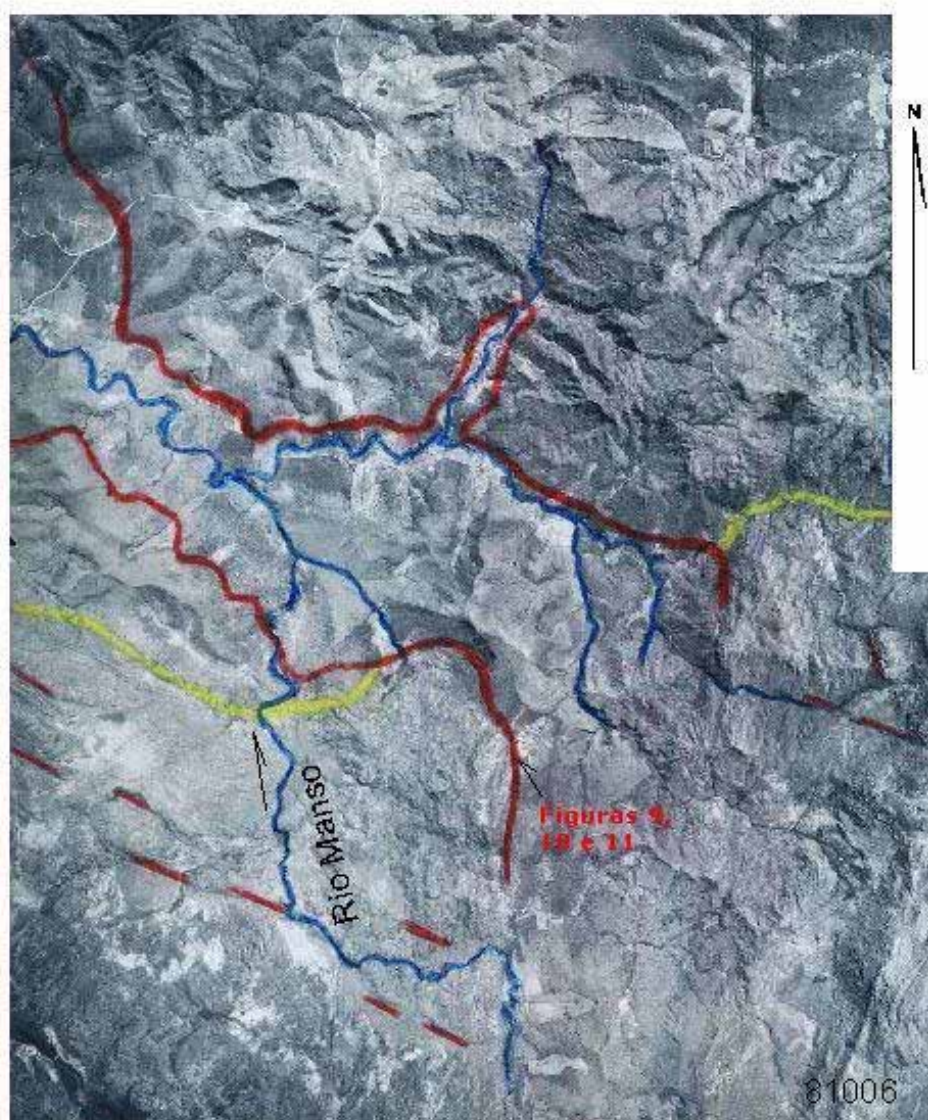
Figura 16 - Foto aérea da USAF - 1965, escala de 1:60.000, cobrindo parte da área do Vale Glacial do Rio Manso e áreas adjacentes. As linhas vermelhas descontinuas marcam os principais lineamentos estruturais e como pode ser observado, cortam apenas os quartzitos e não os tilitos. As linhas vermelhas contínuas marcam os contatos entre quartzitos e tilitos, enquanto as linhas amarelas marcam os contatos entre os quartzitos das formações Duas Barras e Sopa-Brumadinho.
