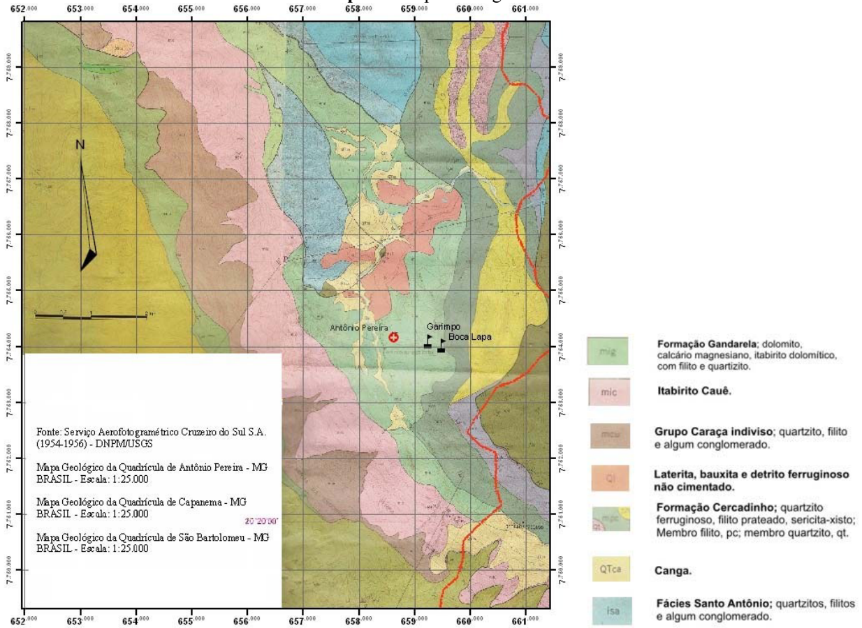
Mapa 1 – Mapa Geológico
